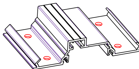
SF300-TOP - THERMAL
