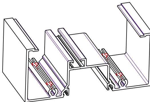
SF300-PROFILE - THERMAL
